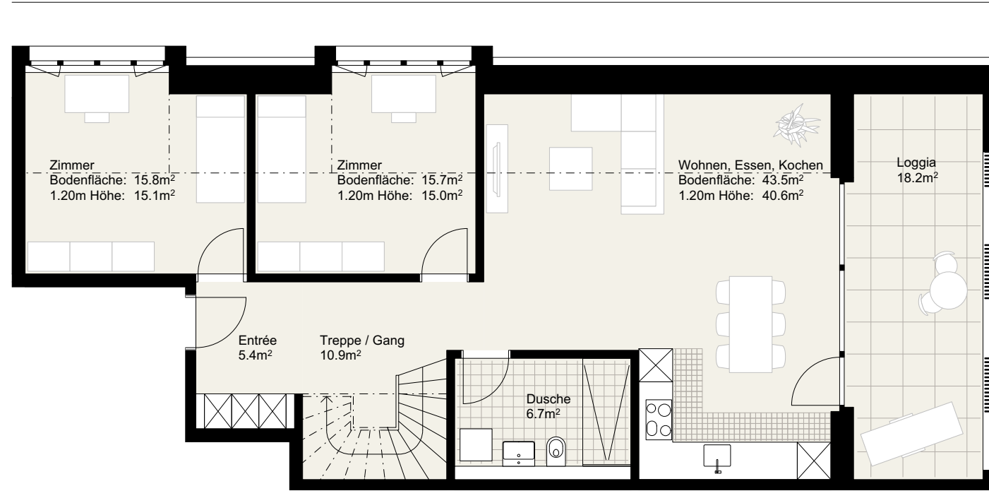
1. Dachgeschoss 1:100
