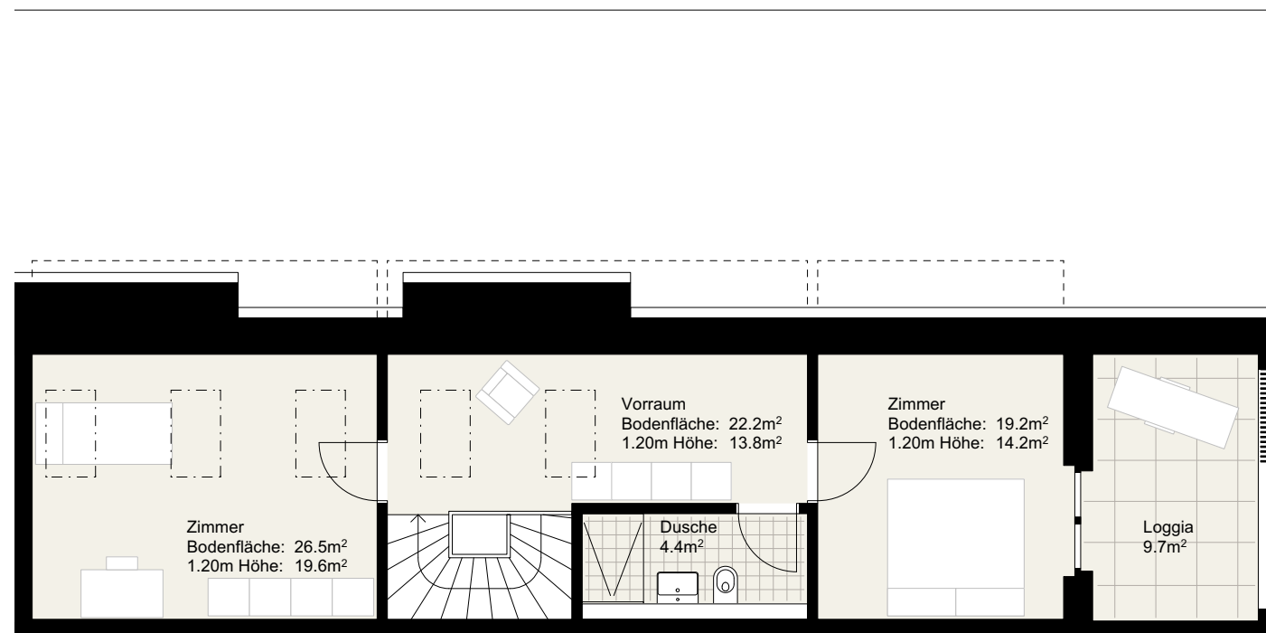
2. Dachgeschoss 1:100
