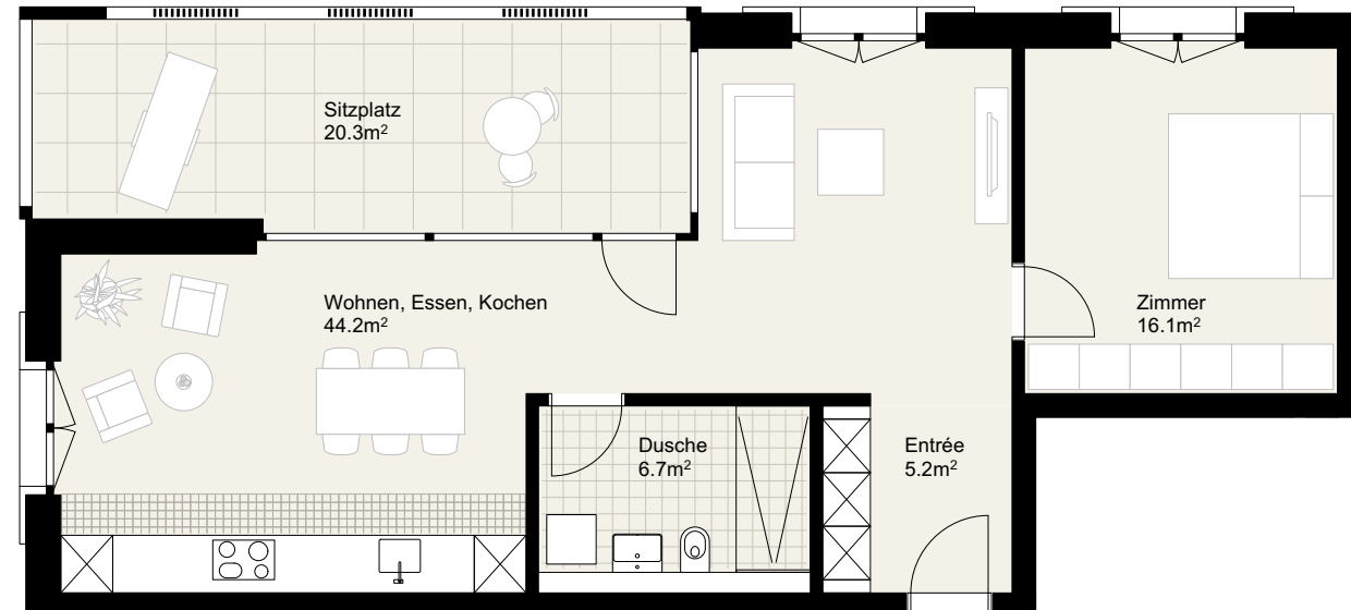
2.5 Zimmer Wohnung 1:100 0 1 2 3 Erdgeschoss
