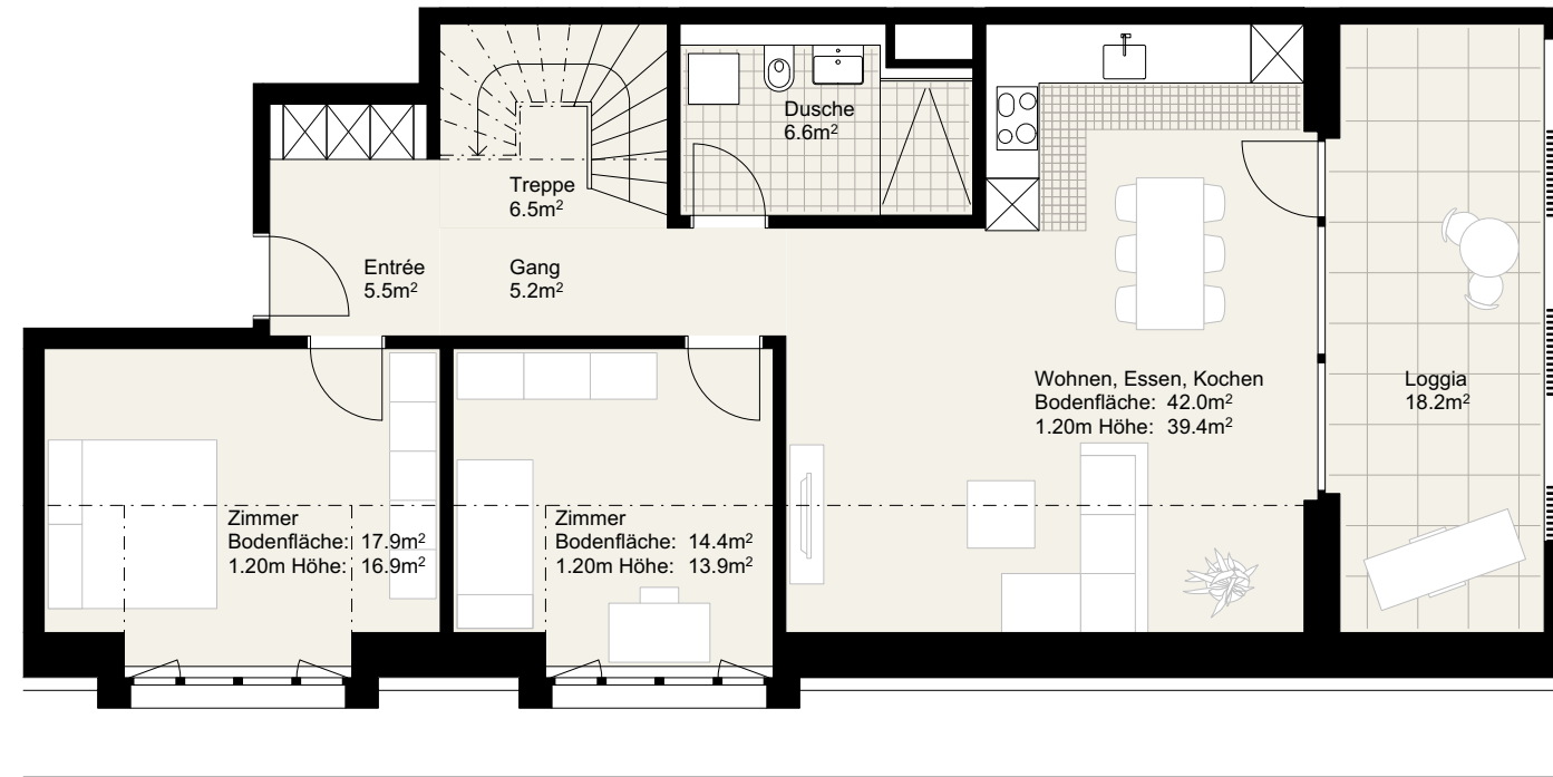
1. Dachgeschoss 1:100 0 1 2 3
