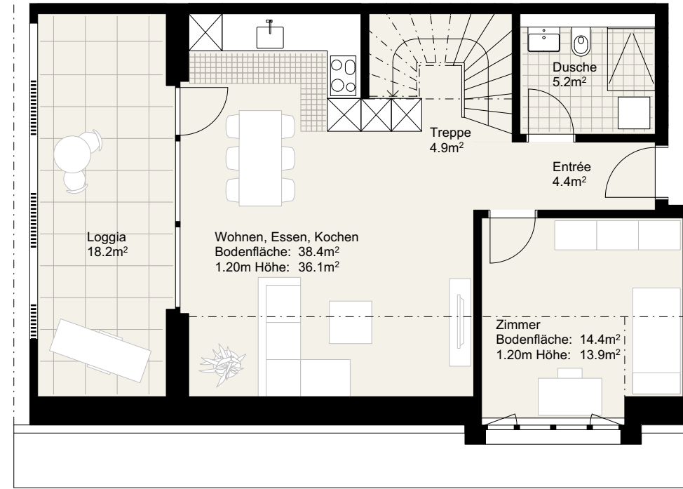
1. Dachgeschoss 1:100 0 1 2 3
