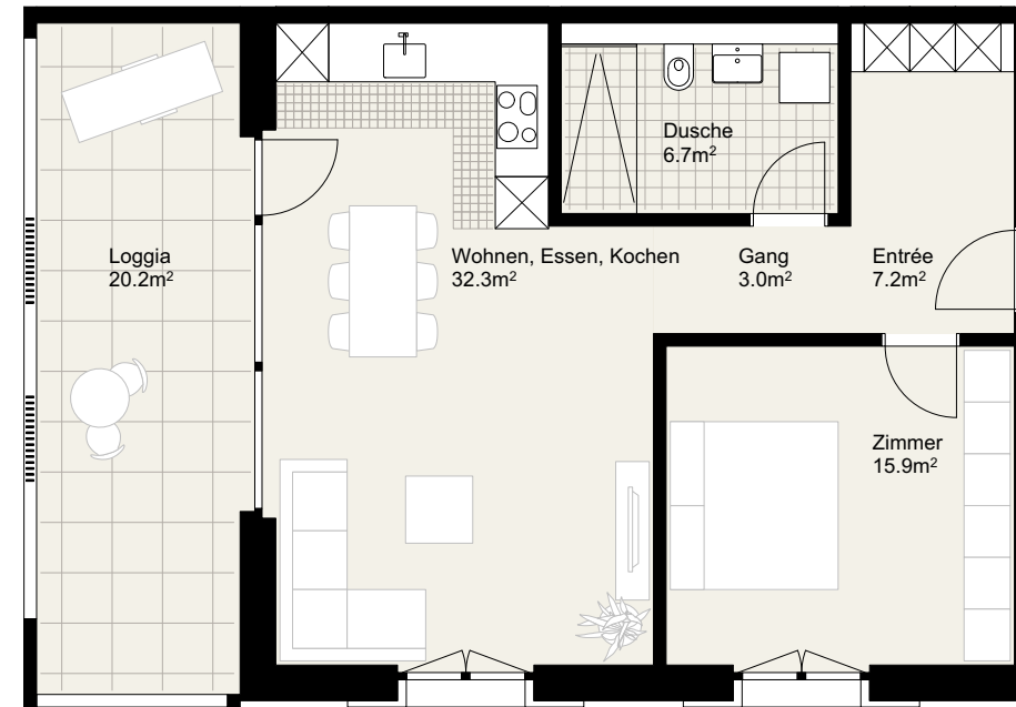
2.5 Zimmer Wohnung 1:100 0 1 2 3 1.Obergeschoss
