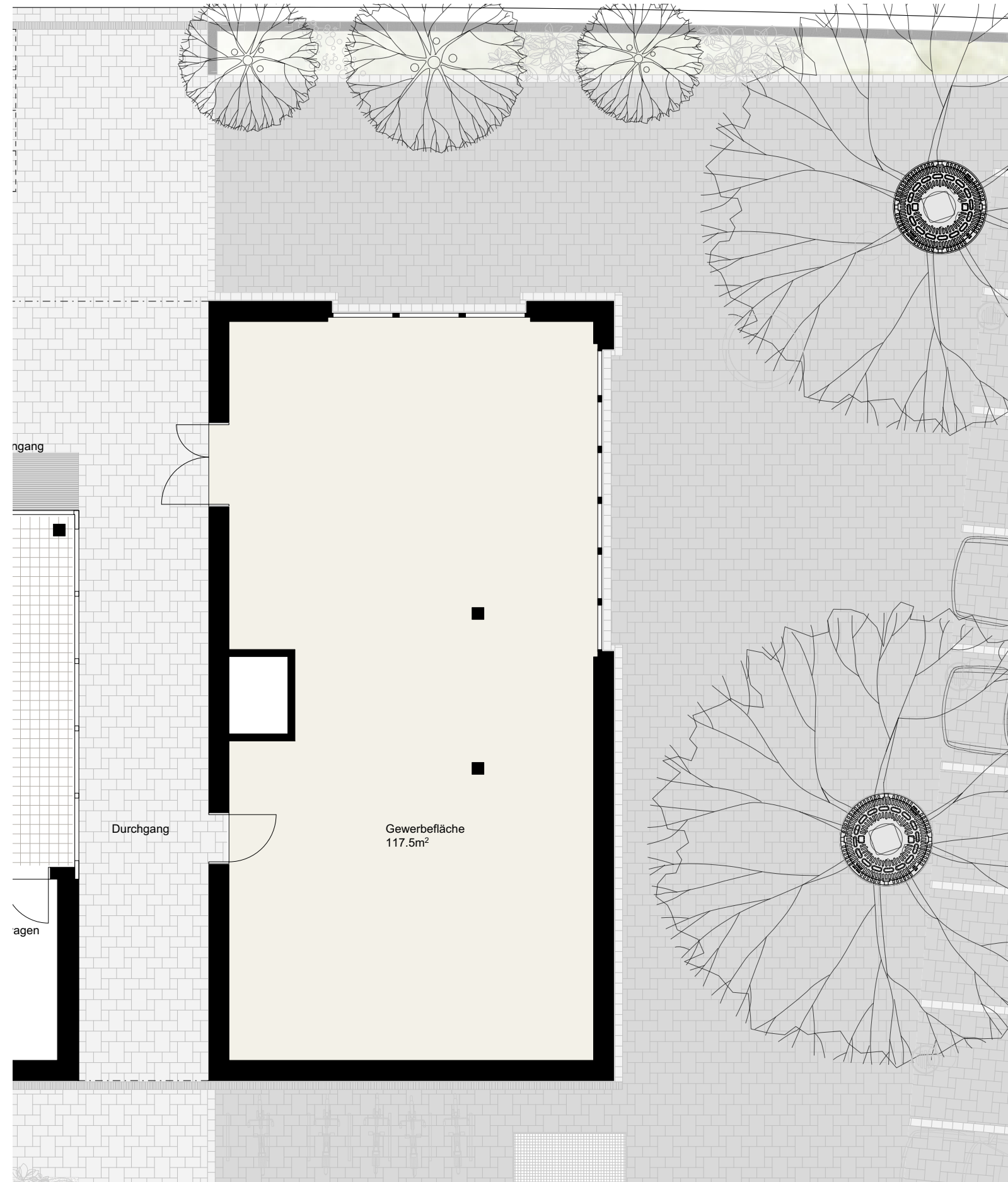
Grundriss 1:100
