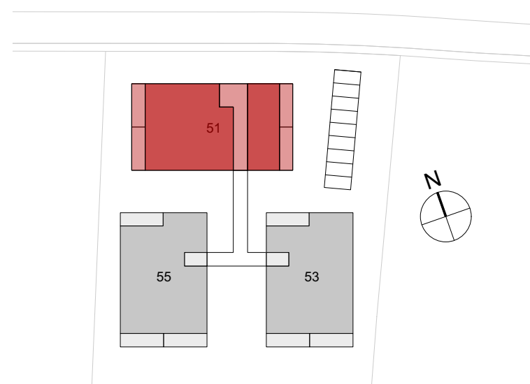
Übersicht Überbauung 1:1000
