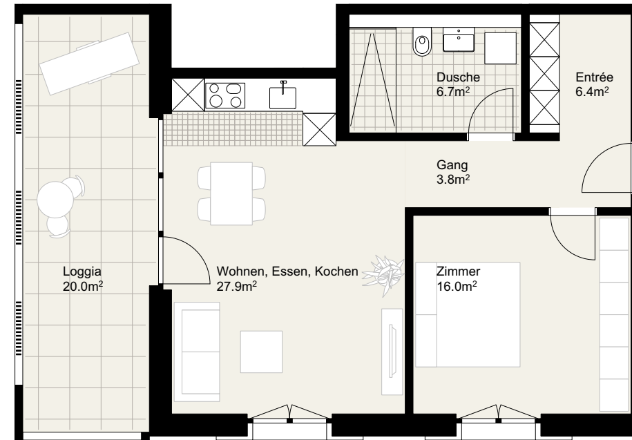
2.5 Zimmer Wohnung 1:100 Erdgeschoss Hochparterre
